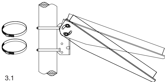
Fig. 3 IT - Staffa di montaggio del pannello solare EN - Solar panel mount bracket FR - Support de montage de panneau solaire
